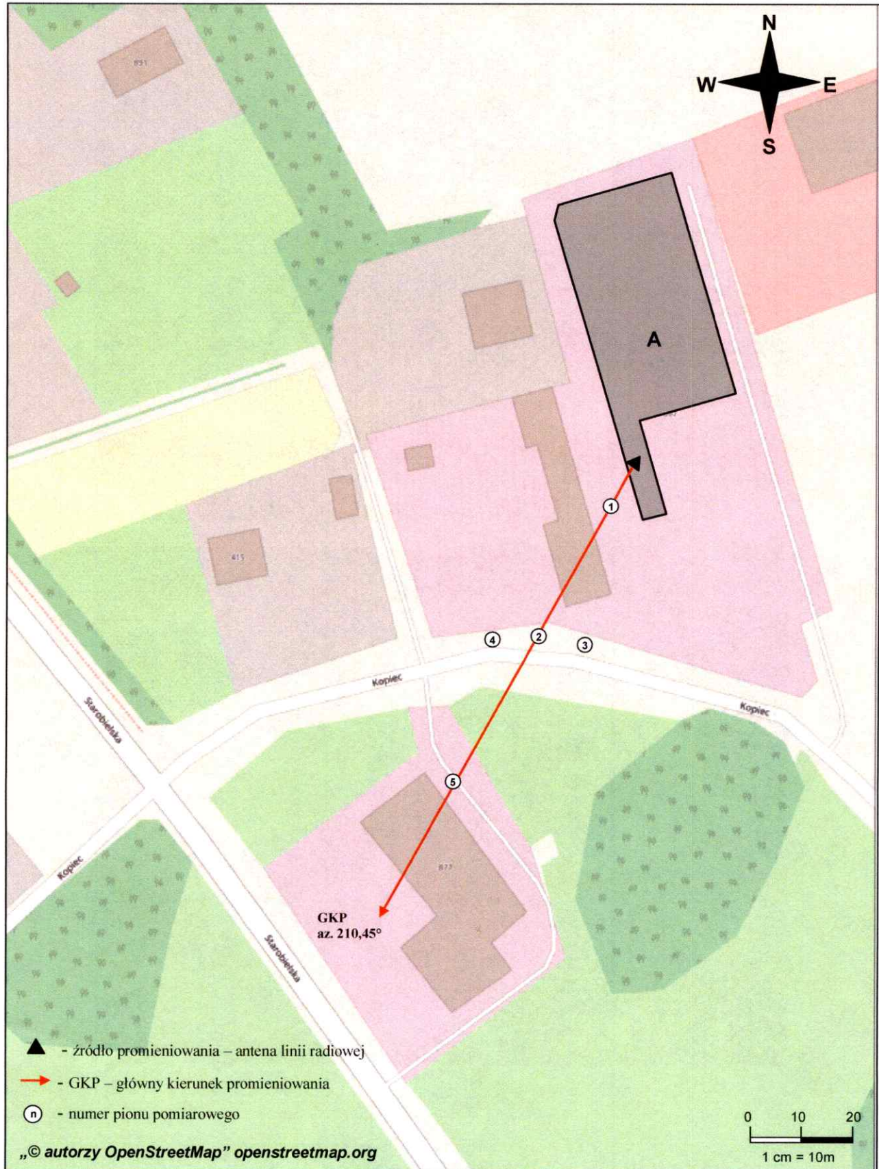
Rys. 1. Usytuowanie punktów i pionów pomiarowych w otoczeniu instalacji radiokomunikacyjnej Stacja Netia JASCB010-JASCM00003 Mazańcowice, ul. Kopiec 1097
